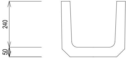
PU1型 - B240-H240
