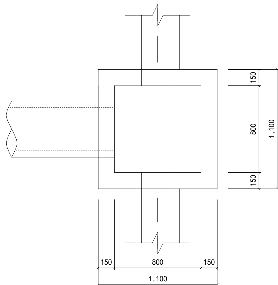
平面圖
